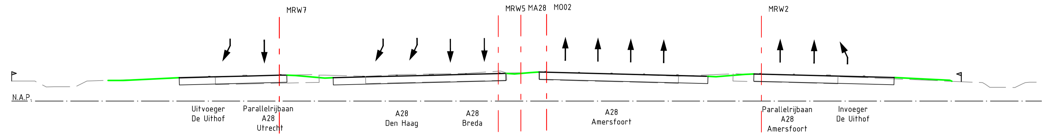
Dwarsprofiel 11 Schaal 1:250
