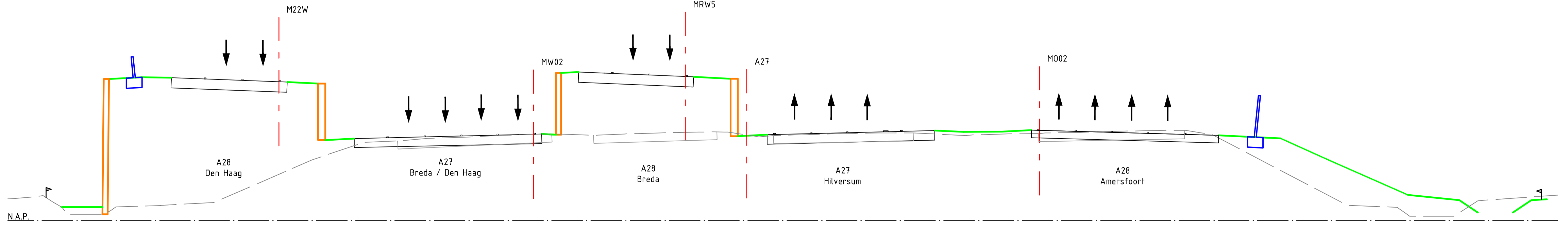
Dwarsprofiel 13 Schaal 1:250
